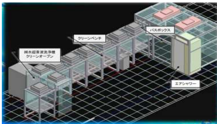
レイアウト
